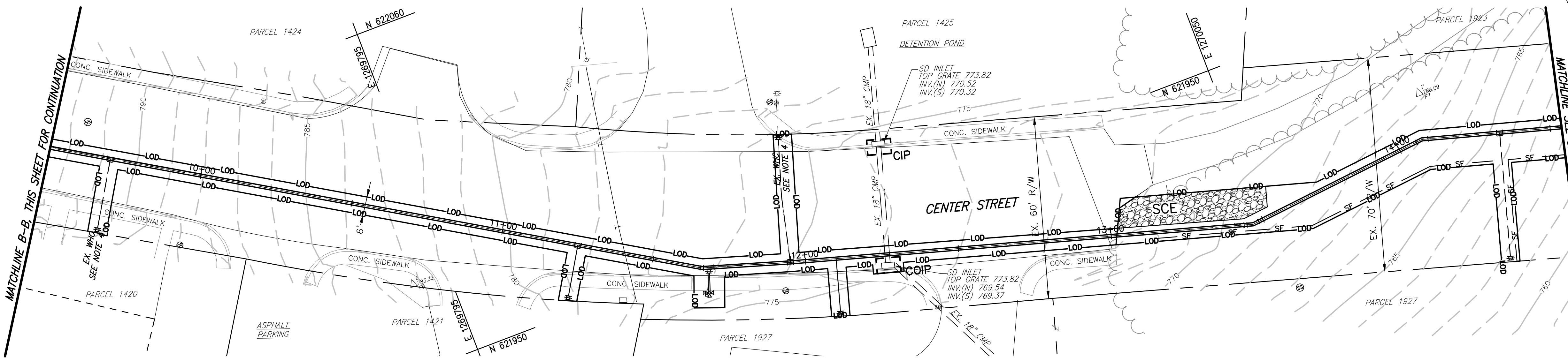
PLAN SCALE: 1"=20'
