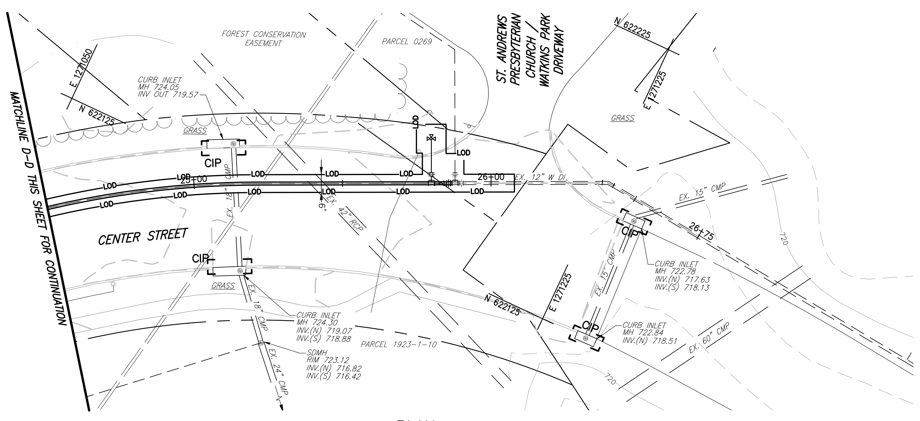
PLAN SCALE: 1"=20'
